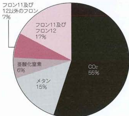
温室効果へのガス別寄与 (1980-1990年)
