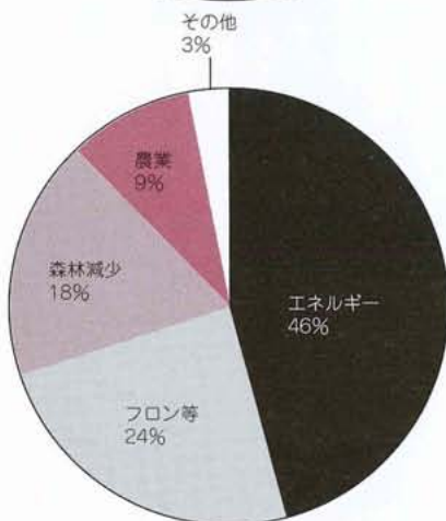
1980年代における人間活動の 地球温暖化への部門別寄与
