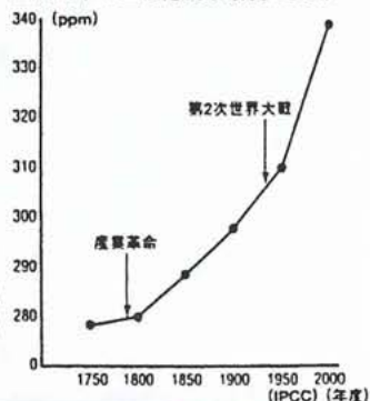
■大気中の二酸化炭素濃度の変化
