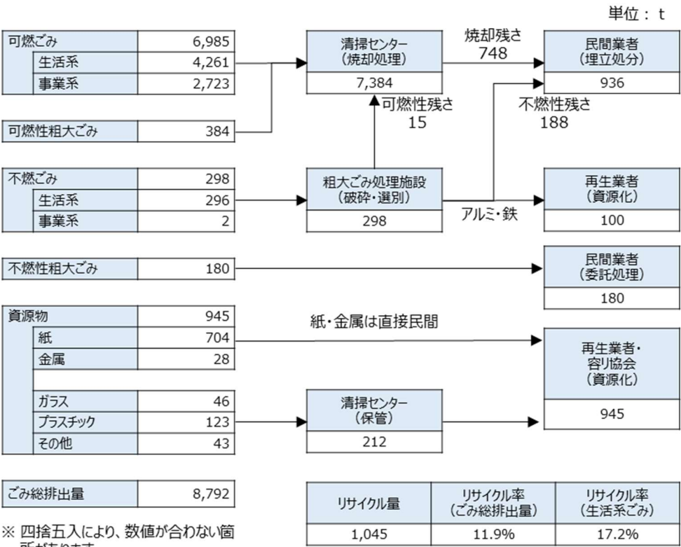
図表3-1-5 ごみ処理の流れ（2022年度（令和4年度）実績）
